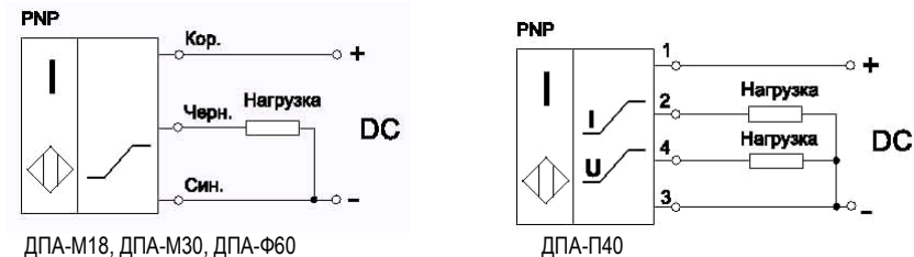
Рис. 2. Схемы подключения датчиков
