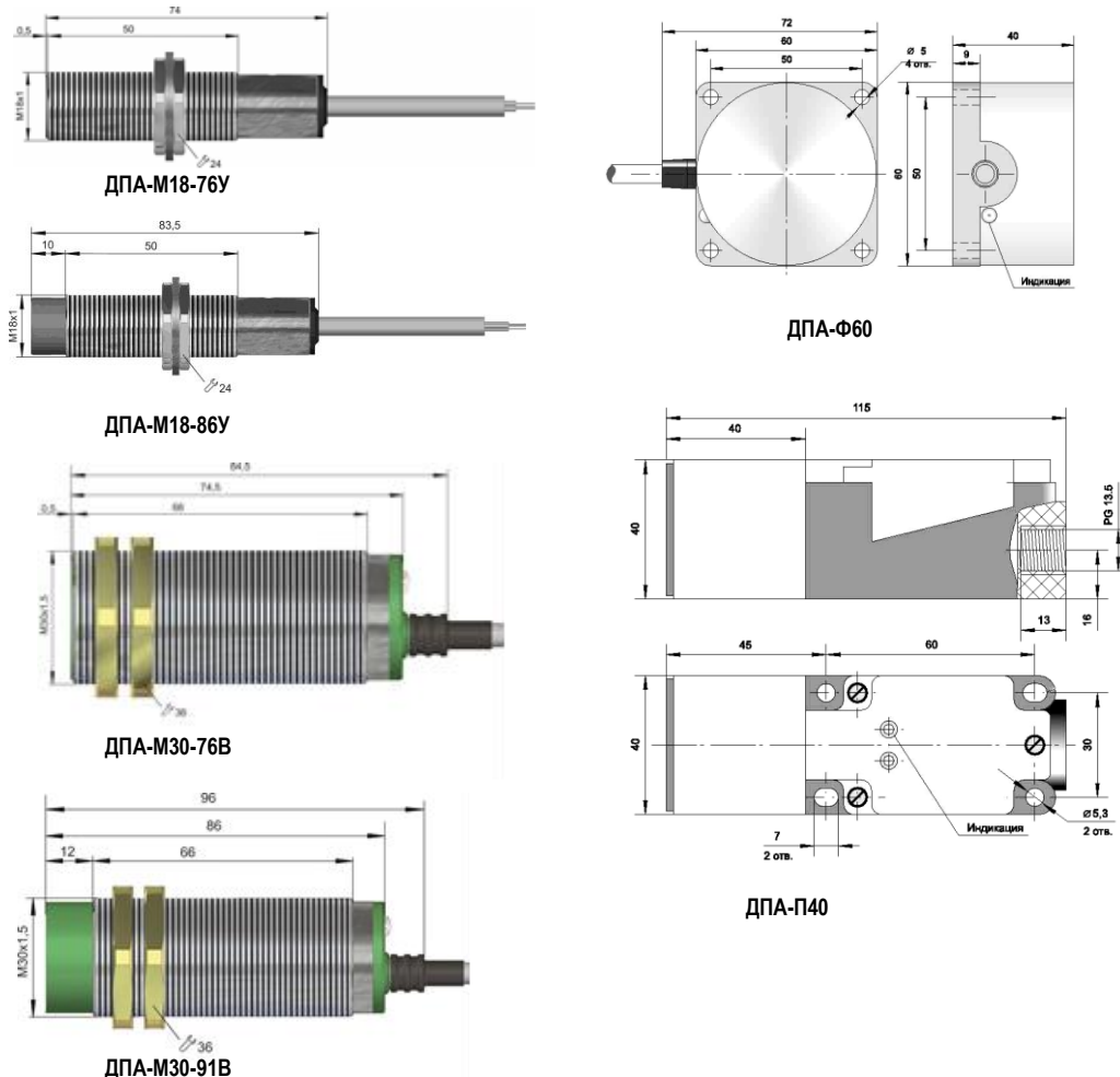
Рис. 1. Габаритные размеры датчиков
