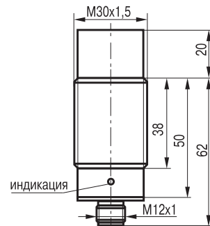
Габаритный чертеж
