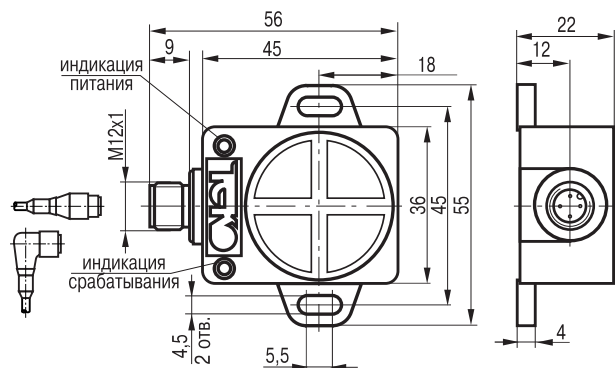
Габаритный чертеж
