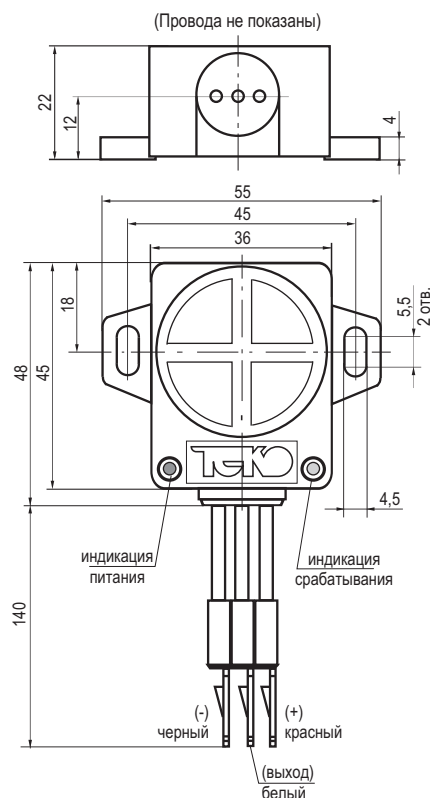
Габаритный чертеж
