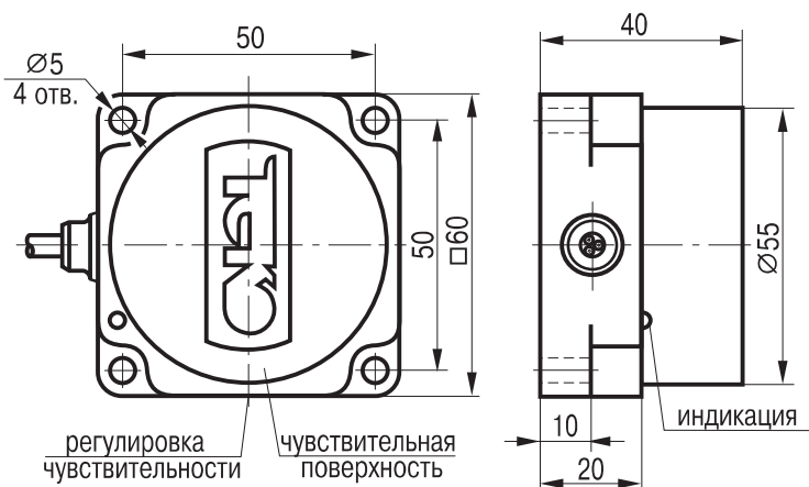
Габаритный чертеж
