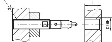
Схема монтажа
