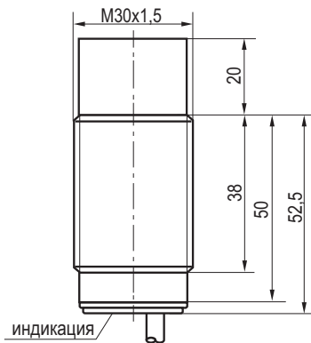
Габаритный чертеж
