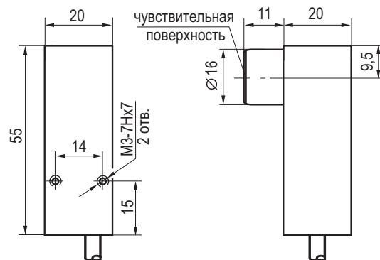
Габаритный чертеж
