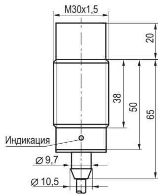
Габаритный чертеж
