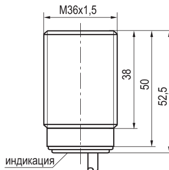
Габаритный чертеж
