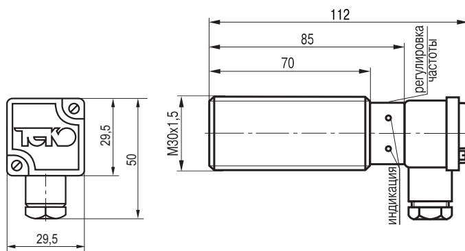
Габаритный чертеж
