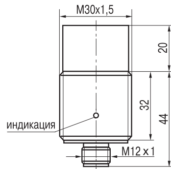
Габаритный чертеж
