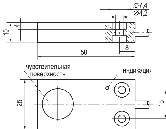
Габаритный чертеж
