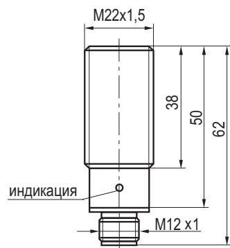
Габаритный чертеж
