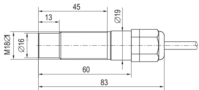
Габаритный чертеж
