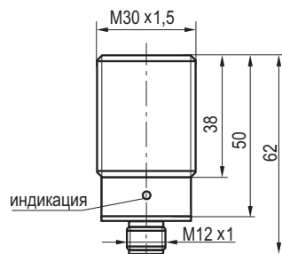
Габаритный чертеж
