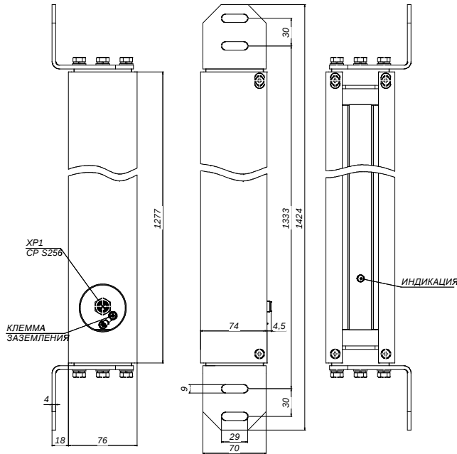
Габаритный чертеж Стойка излучателей (приемников)
