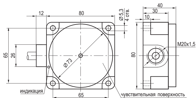
Габаритный чертеж
