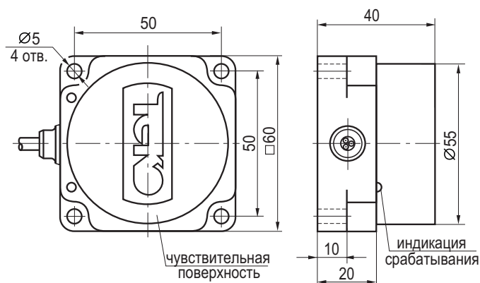
Габаритный чертеж
