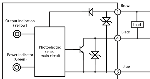
NPN
