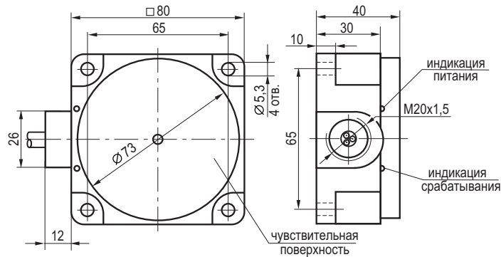
Габаритный чертеж
