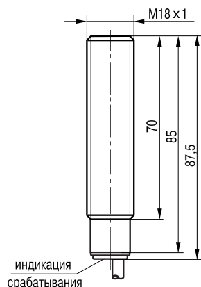
Габаритный чертеж.
