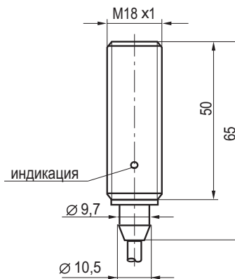
Габаритный чертеж
