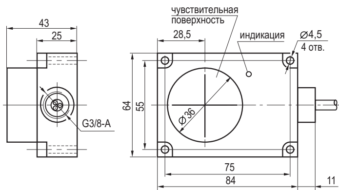
Габаритный чертеж
