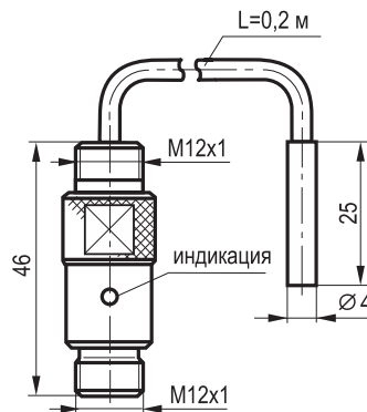
Габаритный чертеж
