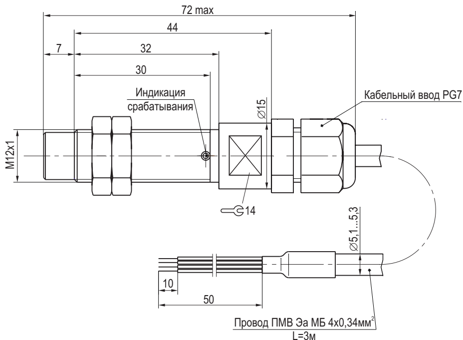
Габаритный чертеж
