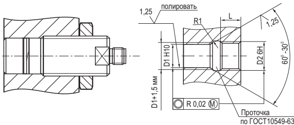
Схема монтажа
