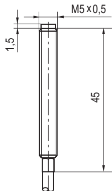
Габаритный чертеж
