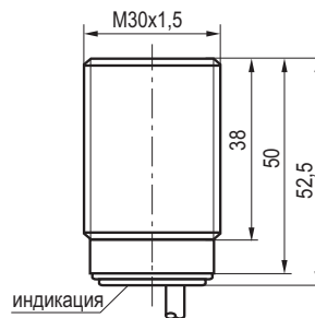
Габаритный чертеж
