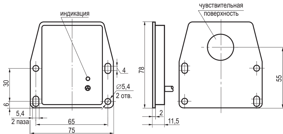
Габаритный чертеж
