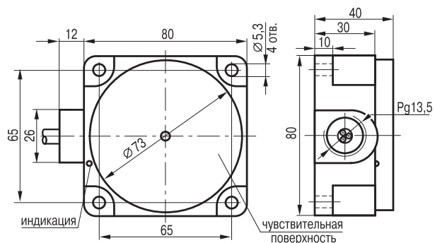
Габаритный чертеж
