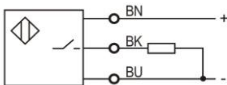
PNP NO
