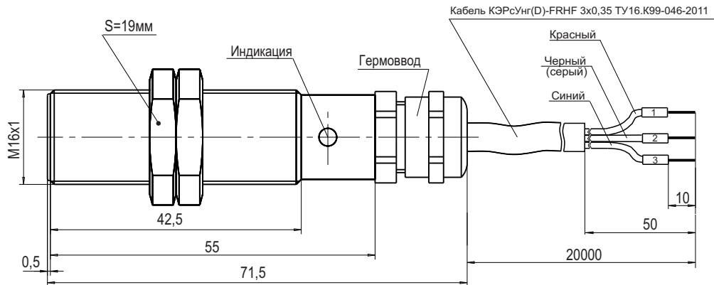
Габаритный чертеж
