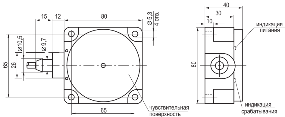
Габаритный чертеж
