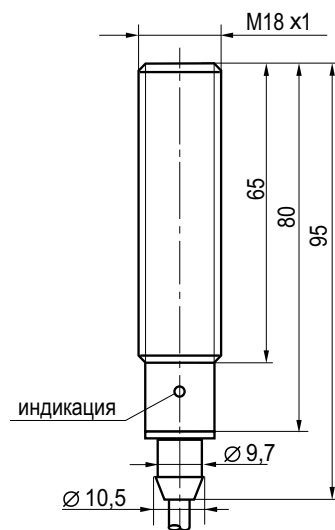
Габаритный чертеж.
