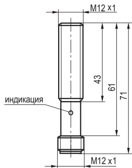
Габаритный чертеж
