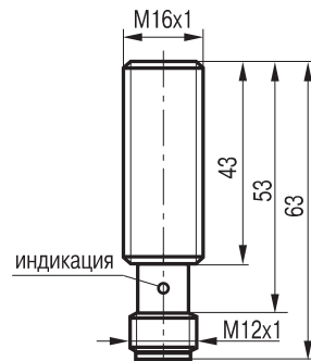
Габаритный чертеж
