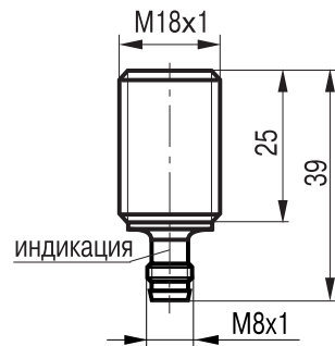
Габаритный чертеж
