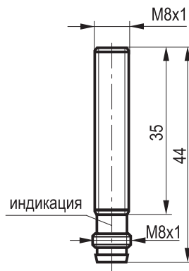
Габаритный чертеж
