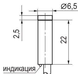
Габаритный чертеж
