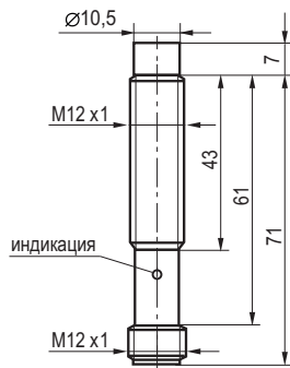
Габаритный чертеж
