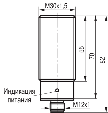
Габаритный чертеж
