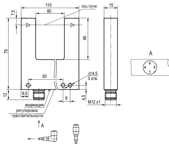
Габаритный чертеж
