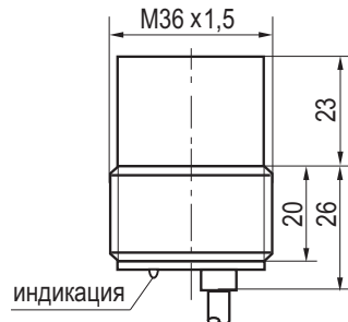
Габаритный чертеж
