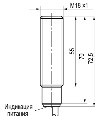
Габаритный чертеж
