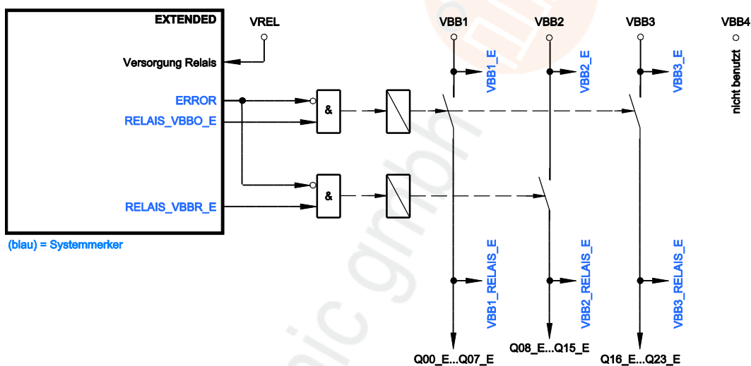
Grafik:Prinzipaufbau der Versorgung und der Relais (Extended-Seite)
