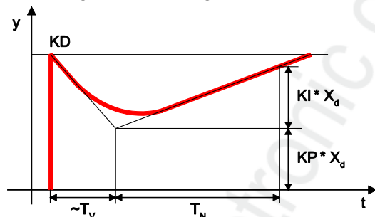
Grafik: Typische Sprungantwort eines PID-Reglers
