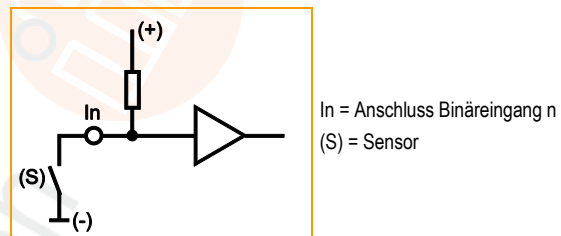
Prinzipischialtung Binäreingang minus-schaltend (BH) für negatives Sensorsignal: Eingang = offen \Rightarrow Signal = High (Supply)
