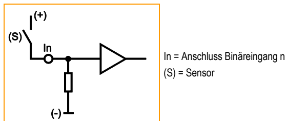
Prinzipischialtung Binäreingang plus-schaltend (BL) für positives Sensorsignal: Eingang = offen \Rightarrow Signal = Low (GND)
