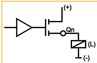
Prinzipschaltung Ausgang plus-schaltend (BH) für positives Ausgangssignal
