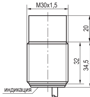
Габаритный чертеж
