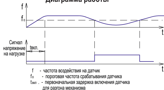
Диаграмма работы
