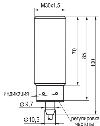
Габаритный чертеж
