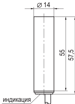
Габаритный чертеж
