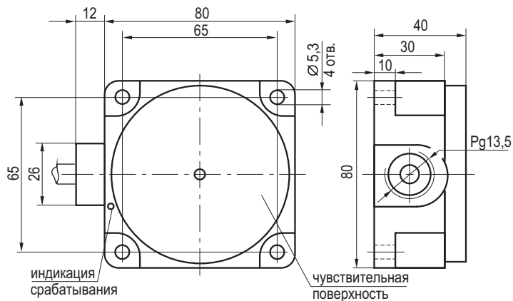
Габаритный чертеж
